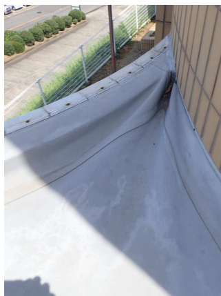
②屋上の劣化 幡豆図書館屋上のシート防水の浮き上がり
