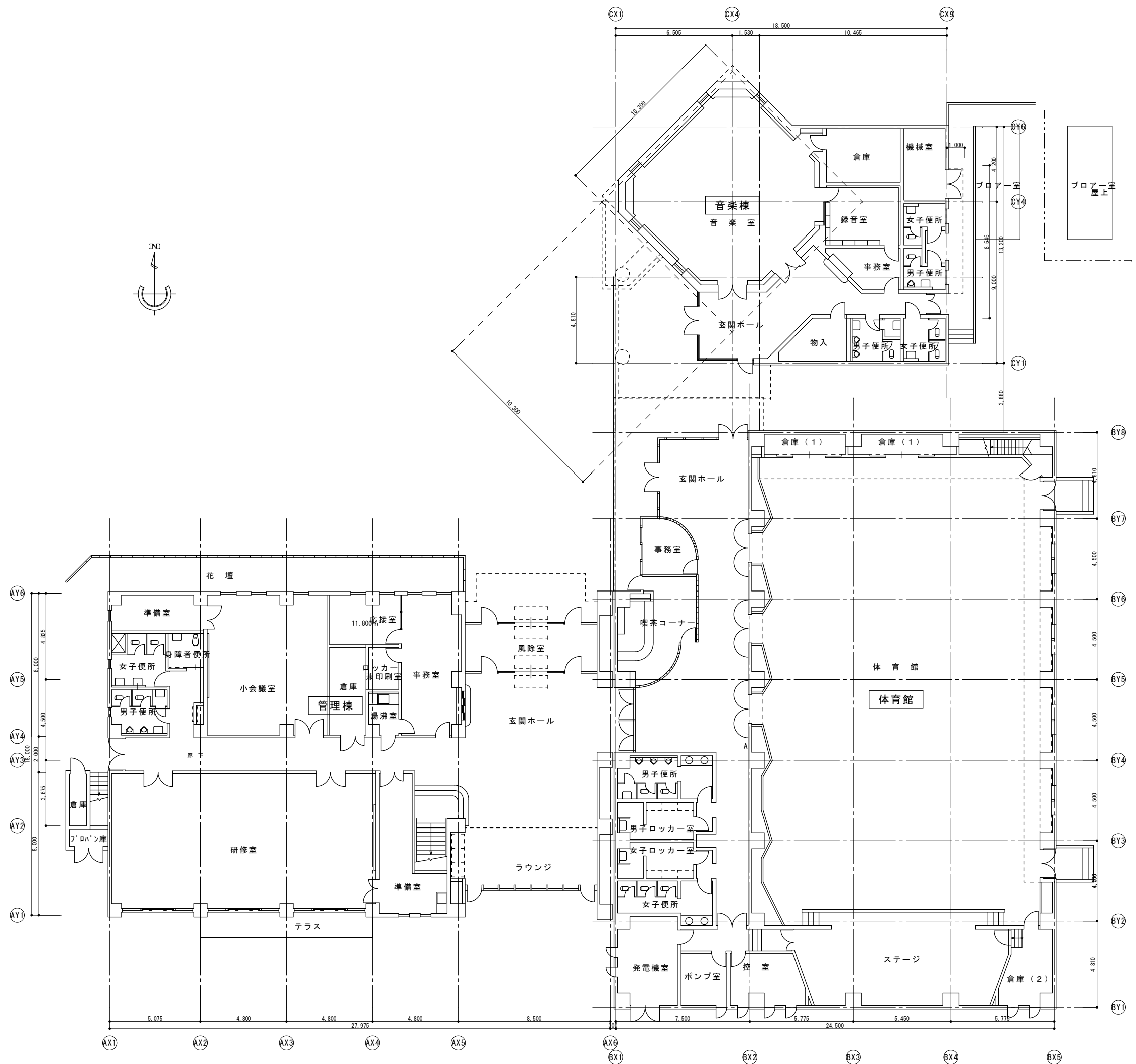
1階平面図 S = 1 / 1 5 0
