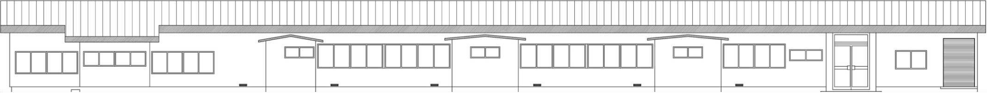
北側立面図 S=1/100
