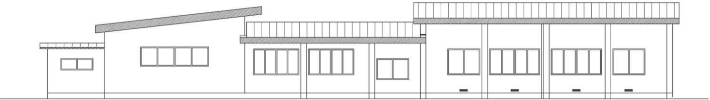
西側立面図 S=1/100
