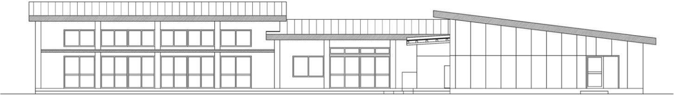
東側立面図 S=1/100
