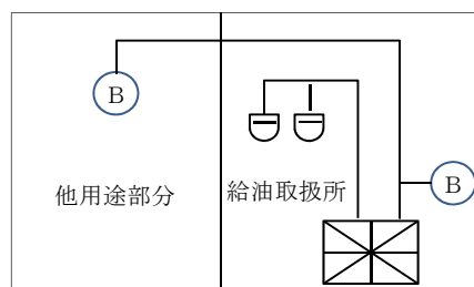
平屋の場合
