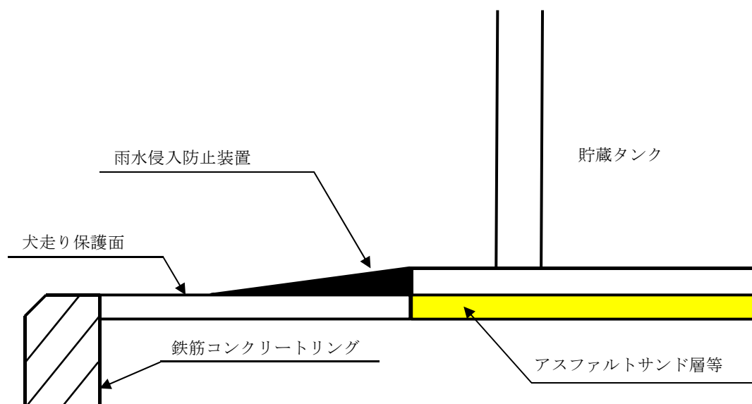
第 1 0 - 3 図 雨水侵入防止措置例 1
