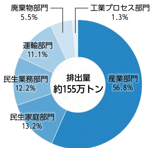
平成29年度市内の二酸化炭素排出量の内訳
