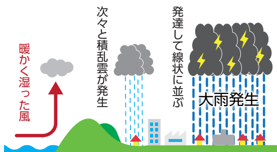
線状降水帯のしくみ
