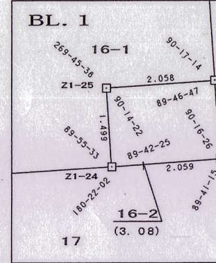
拡大図 1:100
