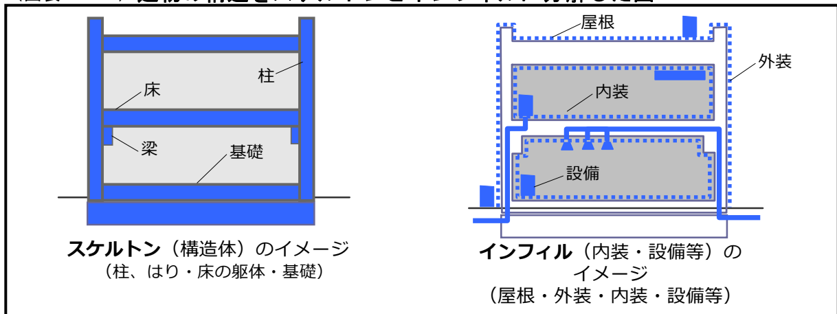
（図表3-1）建物の構造をスケルトンとインフィルに分解した図
