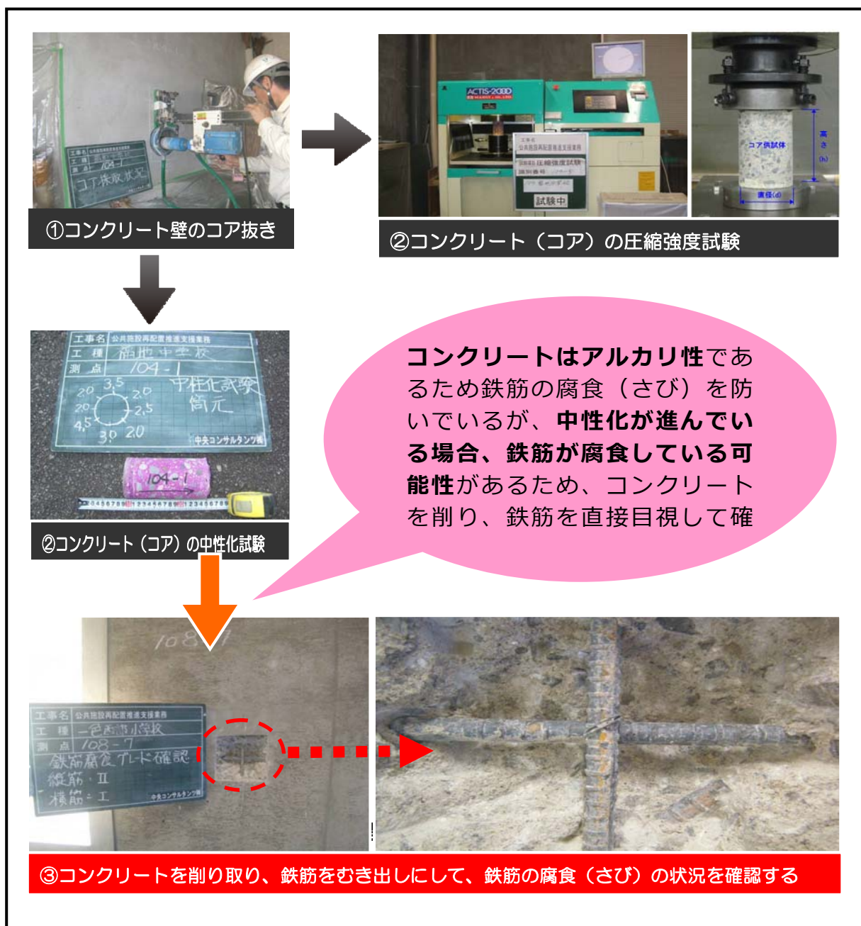
（図表3-2）鉄筋コンクリート造の構造体劣化調査の流れ
