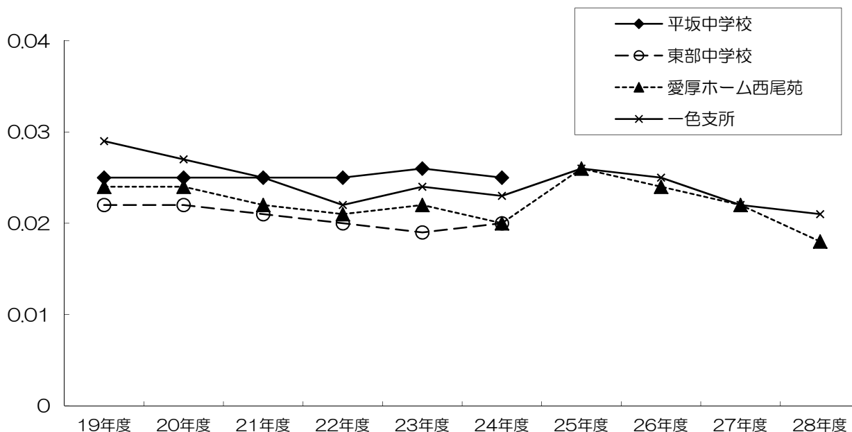
浮遊粒子状物質年平均値の経年変化
